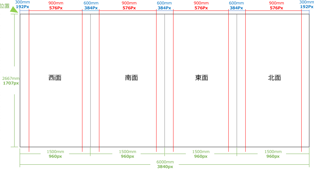
【立面図】
