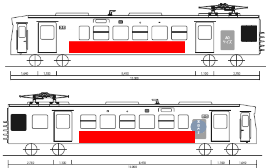
《モ260系 ク160系》
